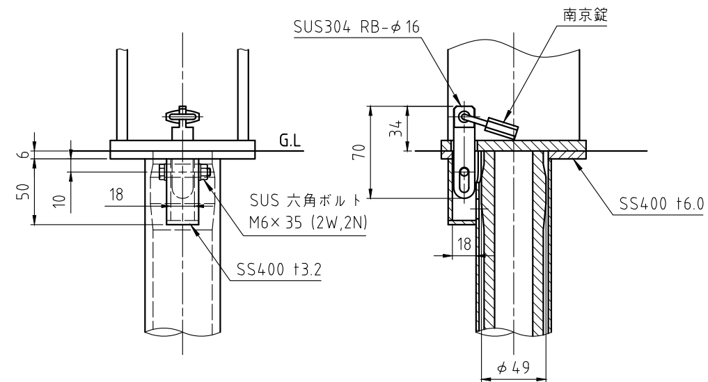
施錠部詳細図 S=1:4
