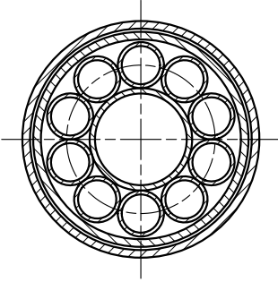
支柱断面詳細図 S=1:4
