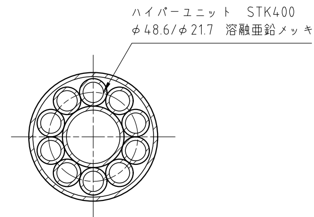
支柱断面詳細図 S=1:3
