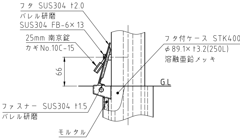
施錠部詳細図 S=1:5
