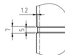
スリット部詳細図 S=1:2
