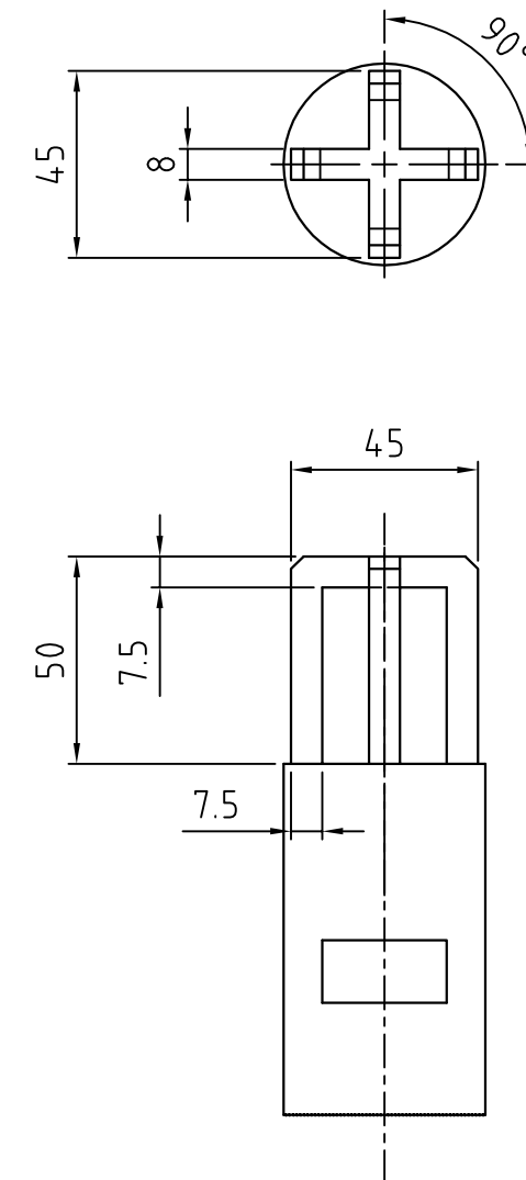
ヘッド詳細図
