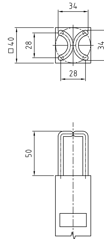
ヘッド詳細図
