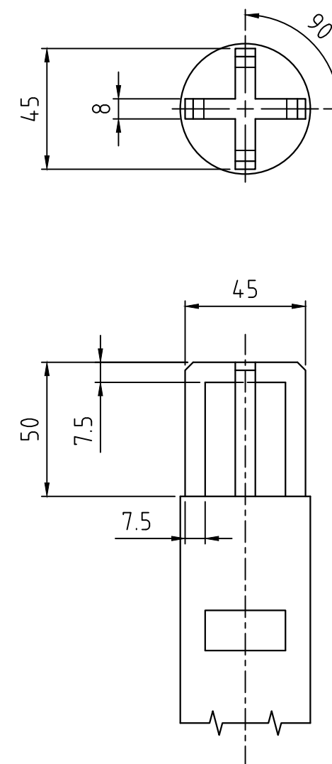
ヘッド詳細図
