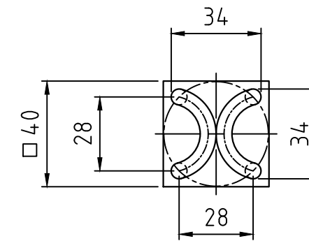
ヘッド詳細図
