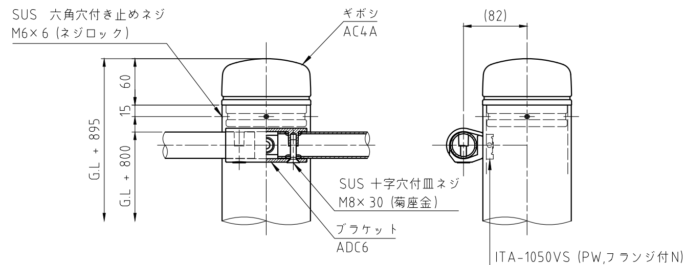
詳細図 S=1:5
