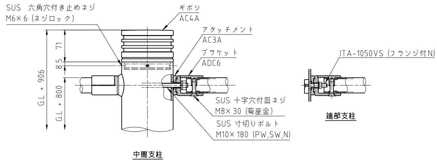
詳細図 S=1:5
