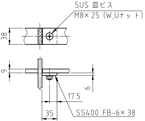
B部 詳細図 S=1:5
