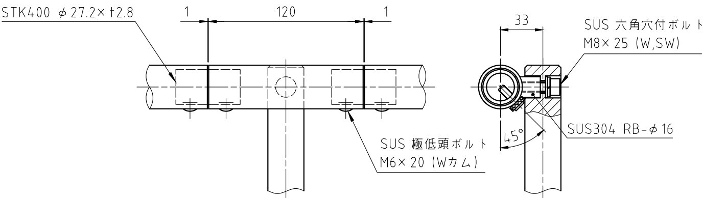
支柱頂部詳細図 S=1:3
