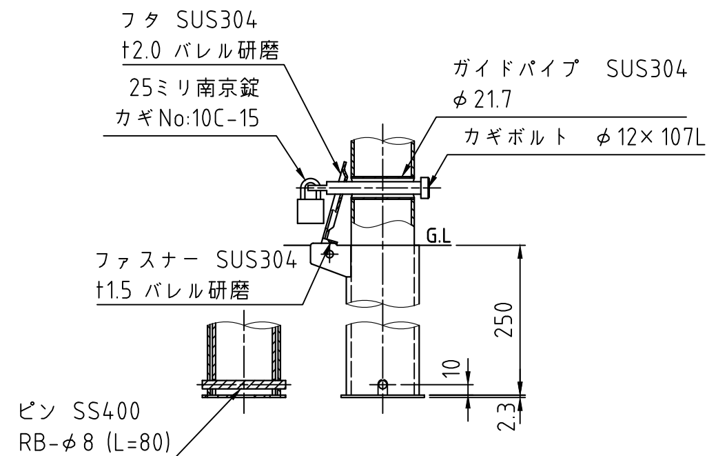
施錠部 / ケース底部詳細図 S=1:5
