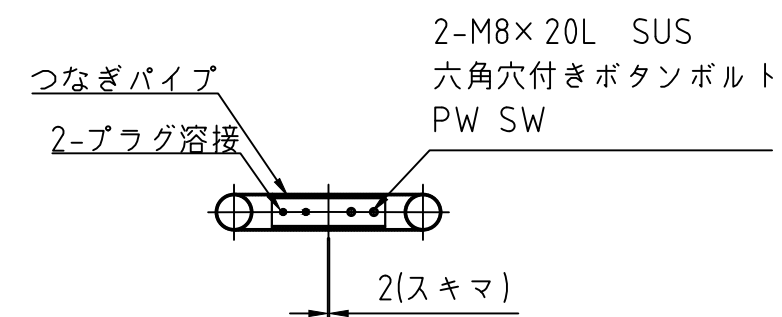
つなぎ部詳細図 S=1:10
