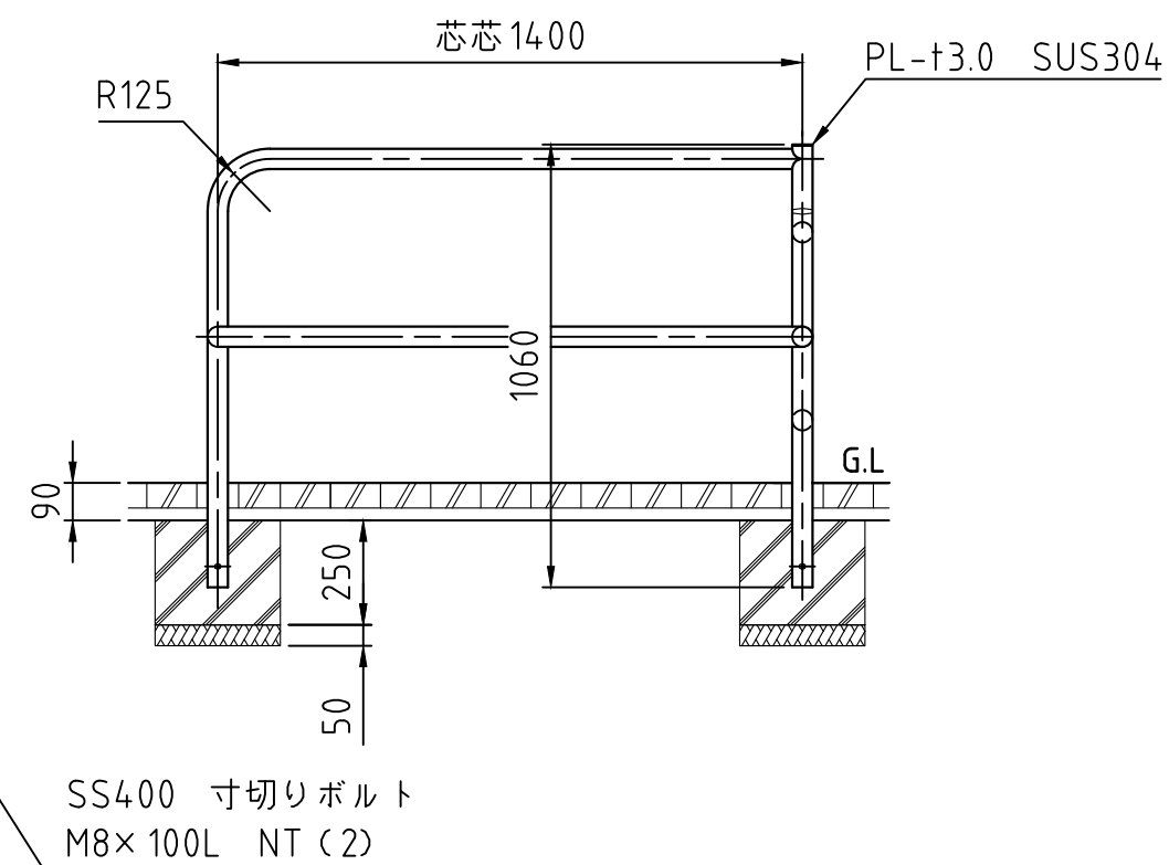
右側面図
